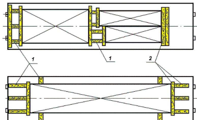
Рисунок 19 – Типовые схемы установки распорных и упорных брусков 1 – распорный брусок; 2 – упорный брусок
