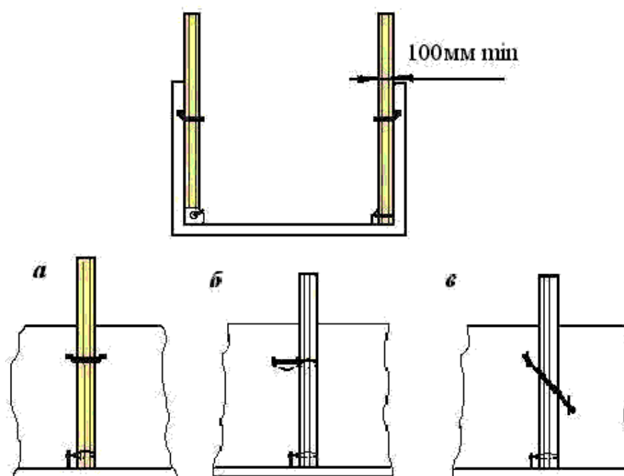
Рисунок 16 – Установка боковых стоек в полувагоне
