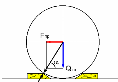
Рисунок 36- Крепление груза от перекатывания упорными брусками
