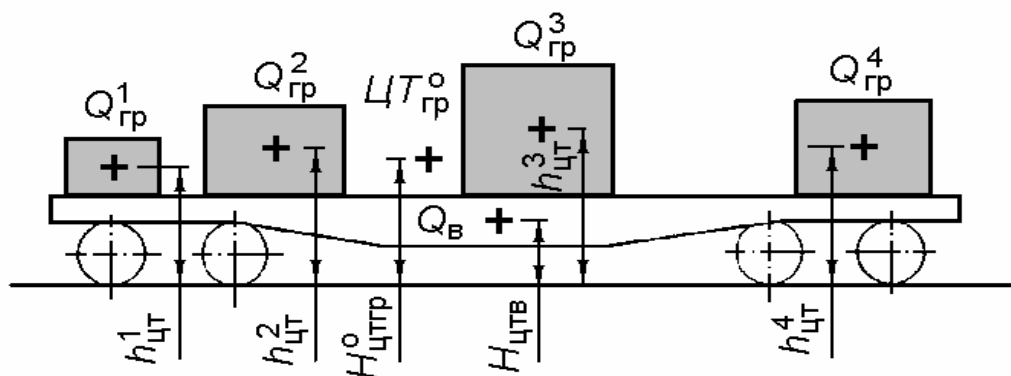
Рисунок 30-Определение высоты центра тяжести вагона с грузом относительно уровня головки рельса
