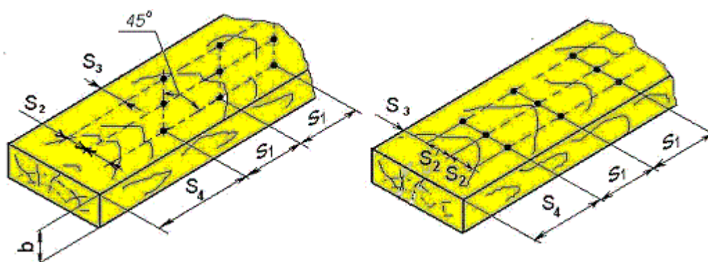
Рисунок 20 – Схемы размещения гвоздей
