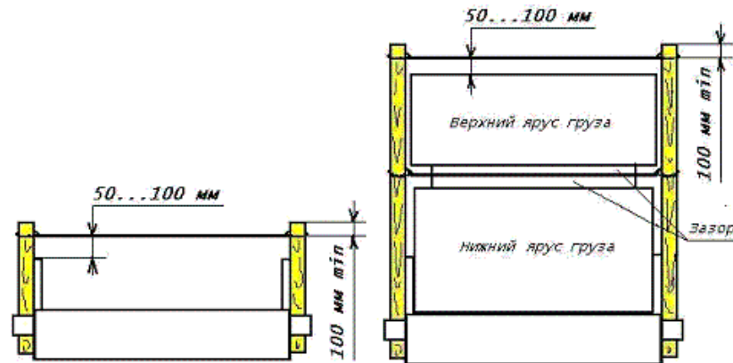
Рисунок 18 – Скрепление стоек на платформе
