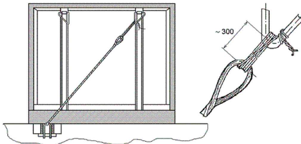
Рисунок 14 – Способ заделки концов проволоки в стяжке.
