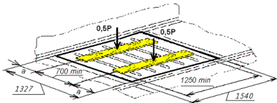
Рисунок 26 – Размещение подкладок на одном люке полувагона
