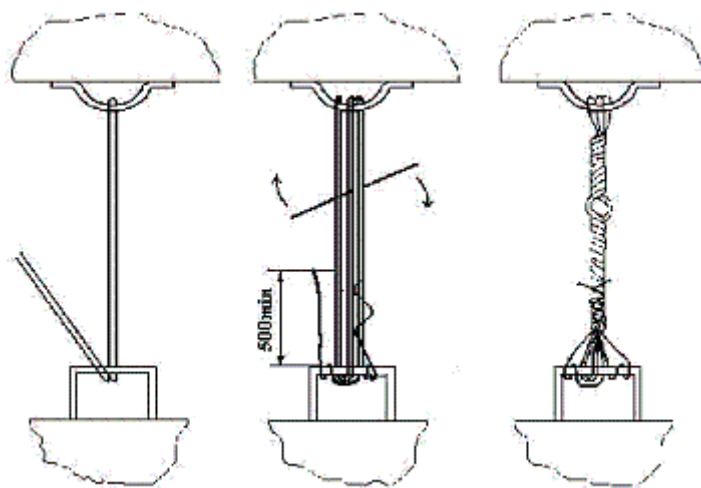
Рисунок 8 – Установка растяжек, обвязок по способу 2
