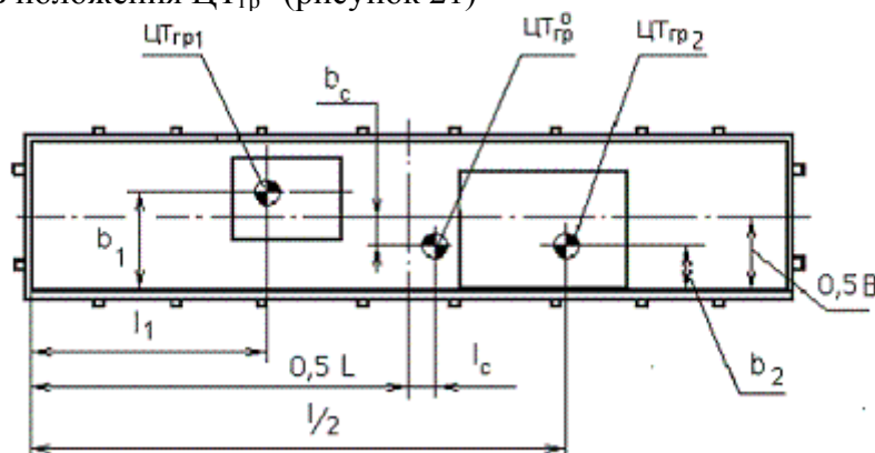
Рисунок 21 – Расчетная схема определения продольного и поперечного смещений общего центра тяжести грузов в вагоне должен выполняться путем расчета величин l_c и b_c по формулам:
