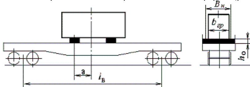
Рисунок 23 - Размещение груза на двух подкладках в пределах базы платформы
