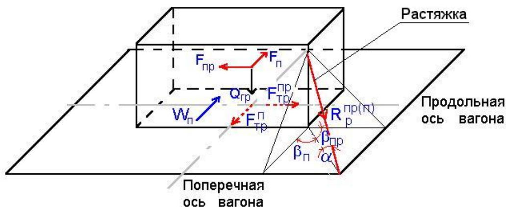
Рисунок 35-Расчетная схема продольных и поперечных усилий в растяжке
