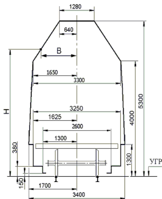
Рисунок 2 – Очертание льготного габарита погрузки
