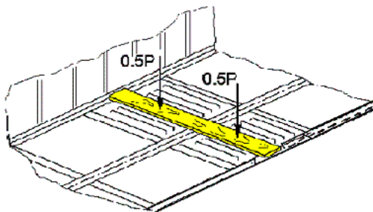
Рисунок 27 – Размещение подкладок на паре люков полувагона
