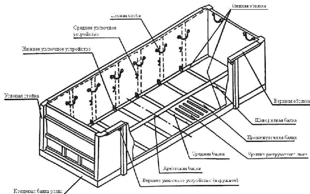
Рисунок 6 – Увязочные устройства универсального полувагона
