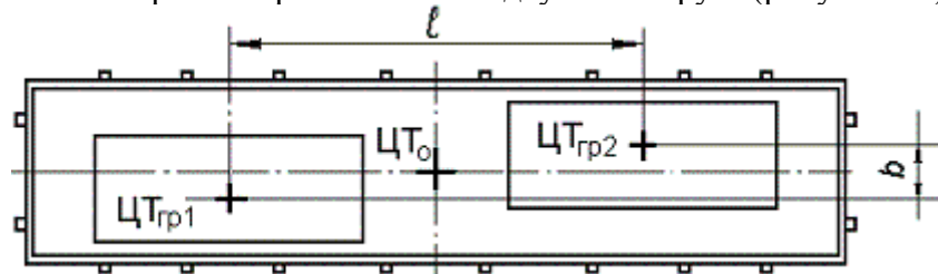
Рисунок 22 - Кососимметричное размещение грузов в вагоне ЦТ гр1 , ЦТ гр2 – центры тяжести грузов; ЦТ 0 – общий центр тяжести вагона с грузом
