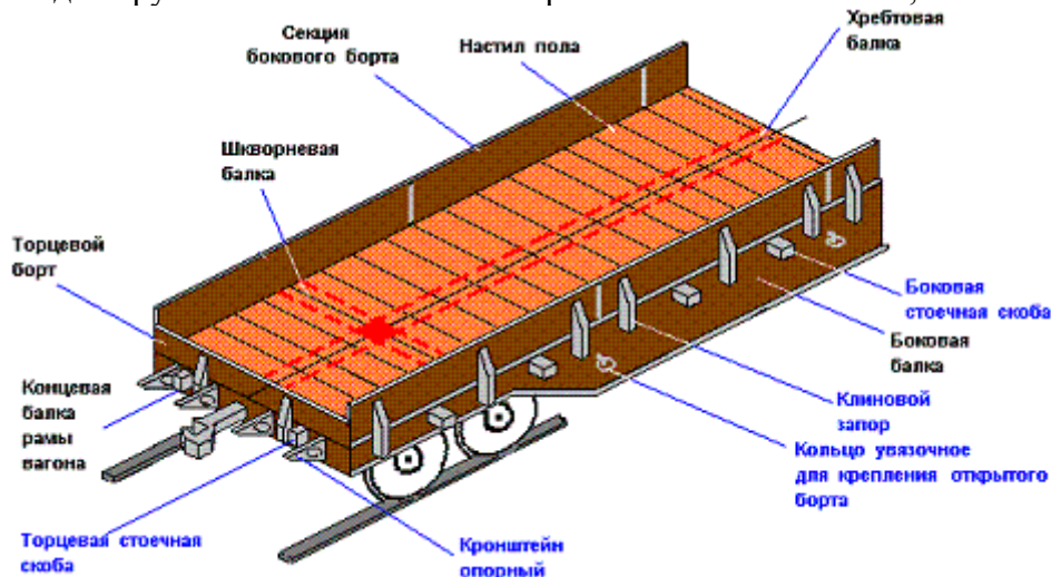
Рисунок 5 – Увязочные устройства универсальной платформы
