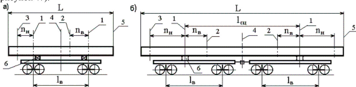
Рисунок 47 – Расчетные сечения длинномерного груза, размещенного а – на одиночном вагоне; б – на сцепе вагонов:
