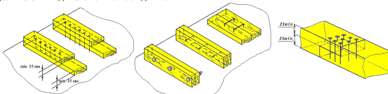
Рисунок 15 – Способы изготовления составных подкладок, прокладок
