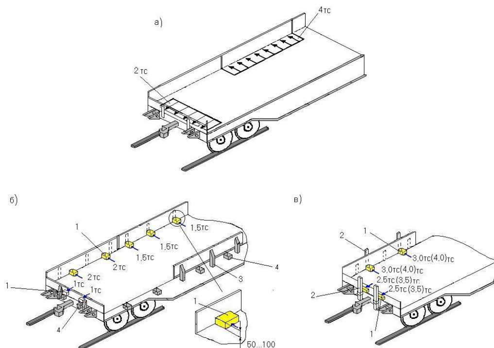
Рисунок 38- Схемы нагружения бортов платформ
