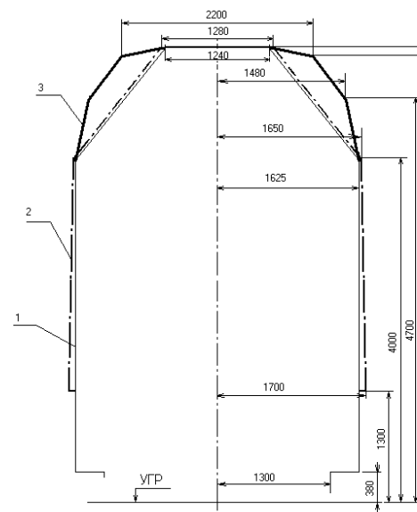
Рисунок 4 - Соотношение очертаний габаритов погрузки
